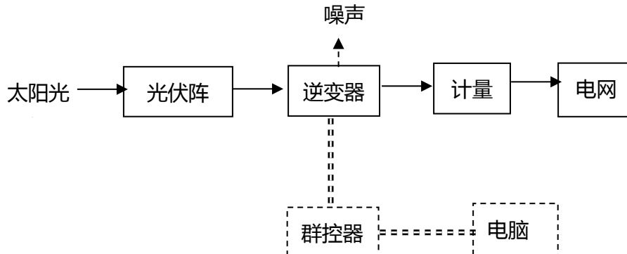
图 2.2-2 运营期生产线工艺流程图
