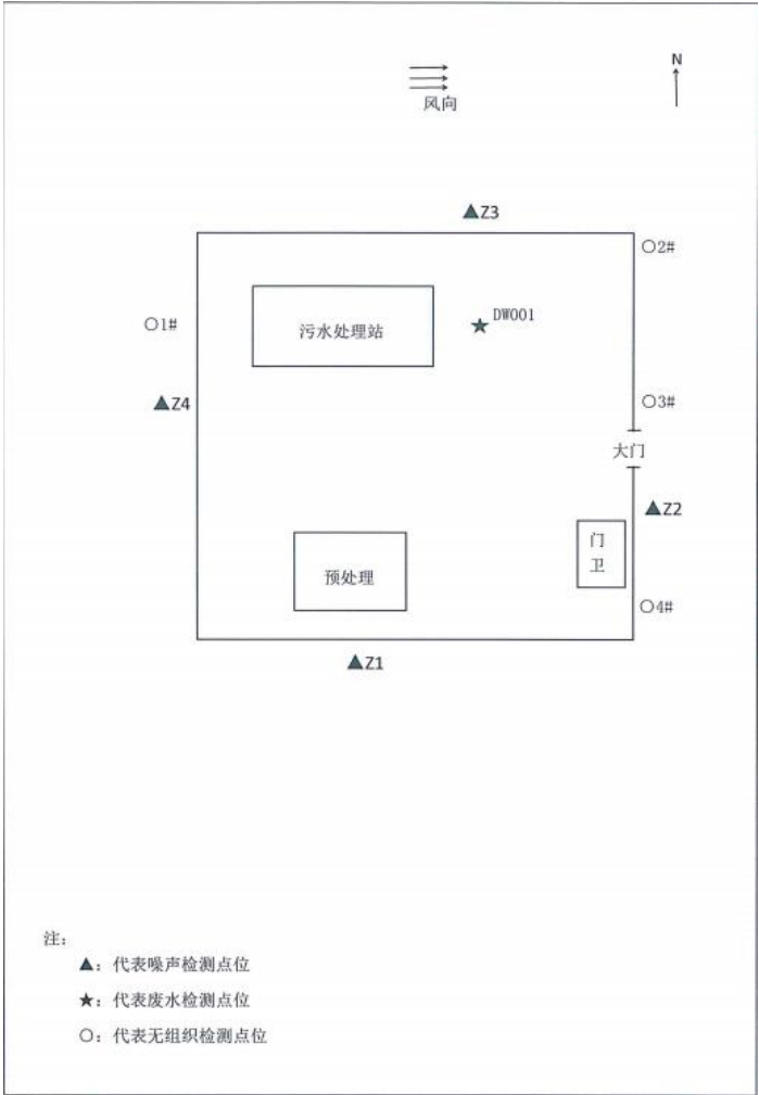
图 6.1-1 项目监测点位示意图（2023 年 6 月 9 日-6 月 10 日）
