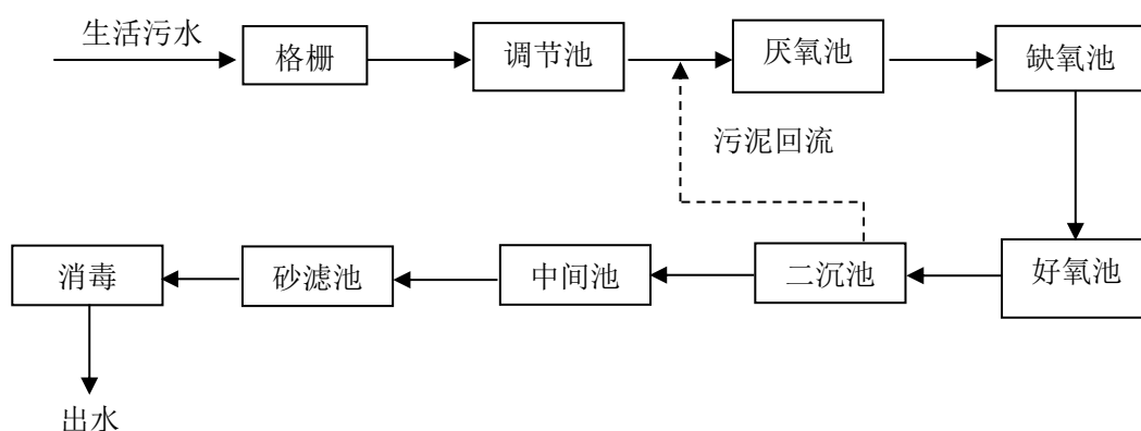
图 2.2-2 邳城镇污水处理厂一期工艺流程及产污环节图
