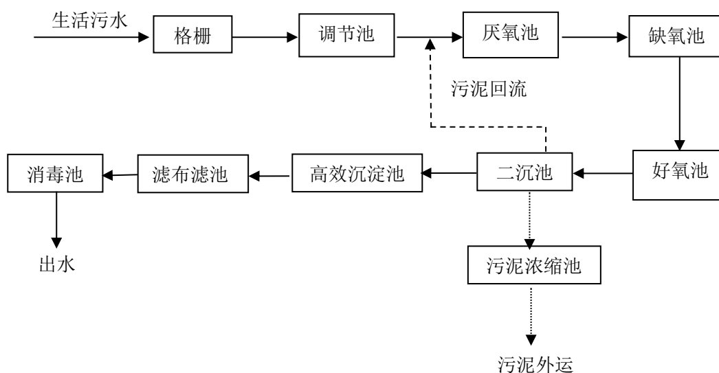
图 2.2-2 占城镇污水处理厂工艺流程及产污环节图
